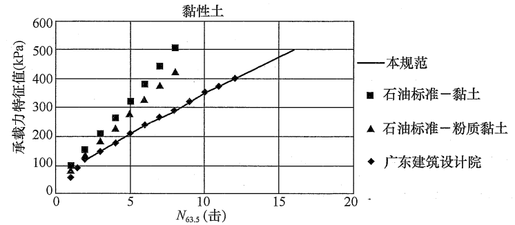
图5 黏性土承载力特征值与 N_{63.5} 关系
