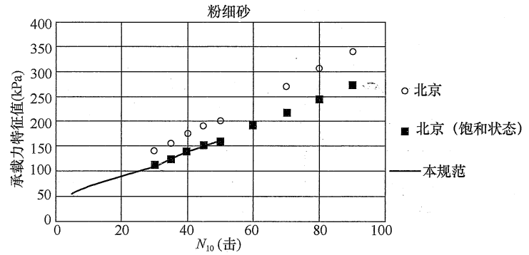
图4 粉细砂承载力特征值与 N_{10} 关系
