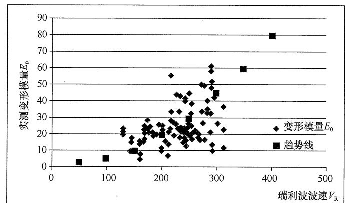
图 16 实测变形模量 E_0 与瑞利波波速 V_R 关系图
