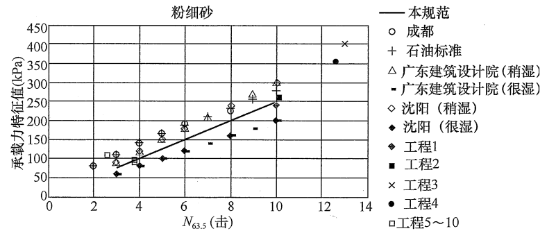
图6 粉细砂承载力特征值与 N_{63.5} 关系
