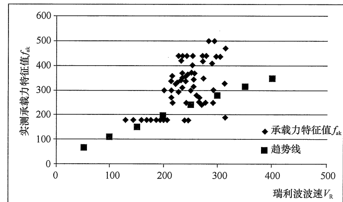
图 15 实测承载力特征值 f_{ak} 与瑞利波波速 V_R 关系图
